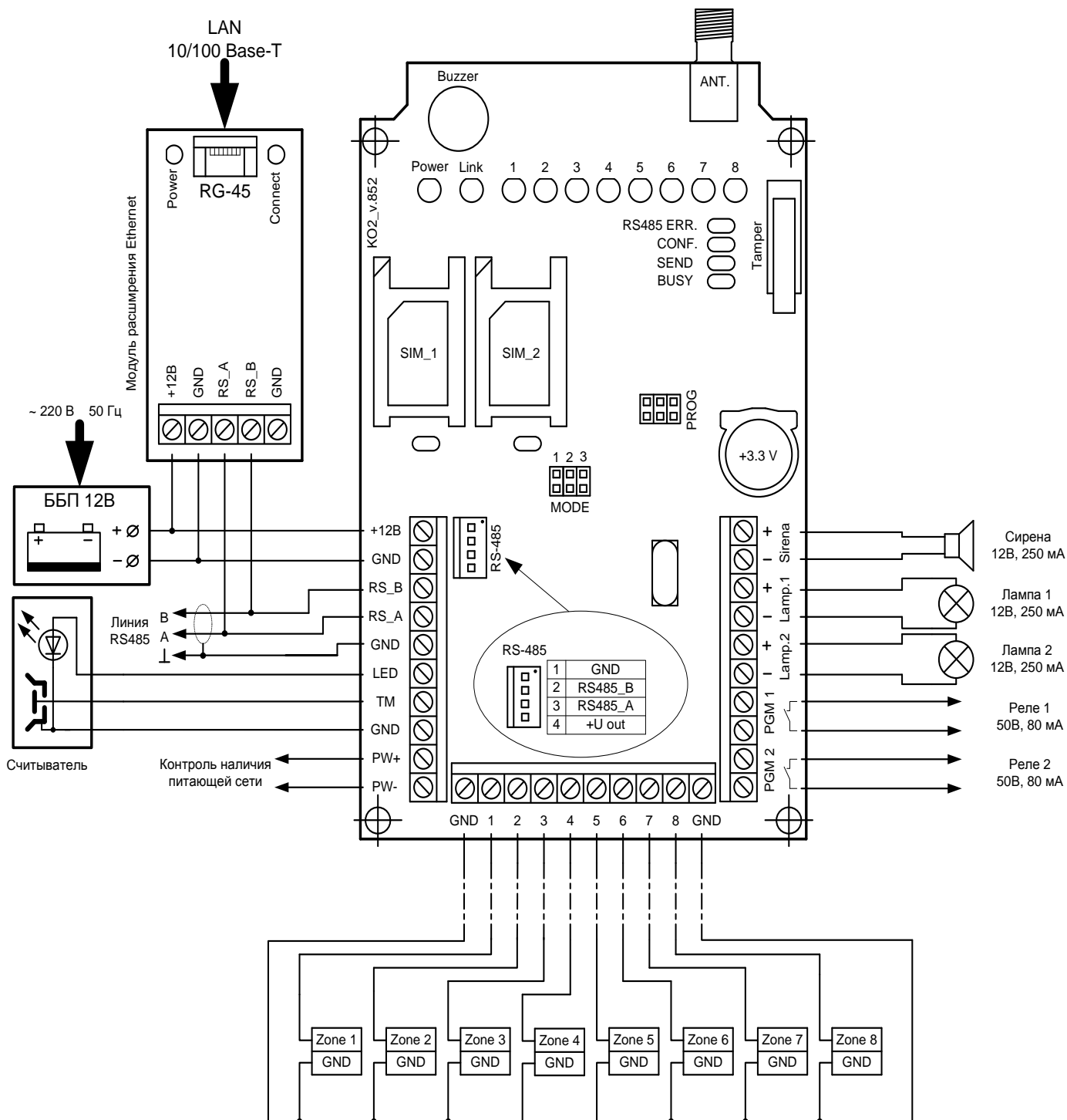
Рисунок 2. Схема подключения прибора.
