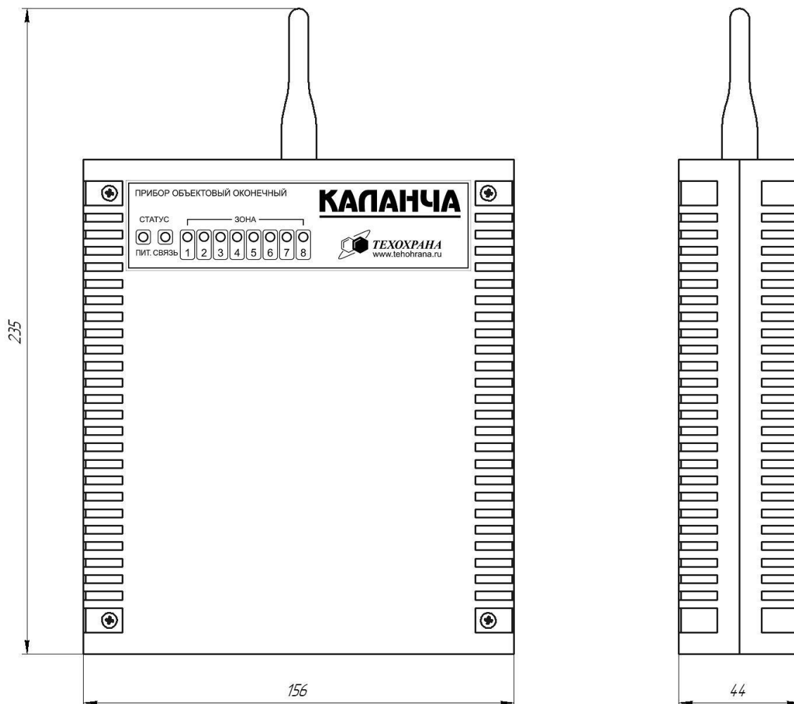
Рисунок 1. Внешний вид и установочные размеры ПОО «КАЛАНЧА»
