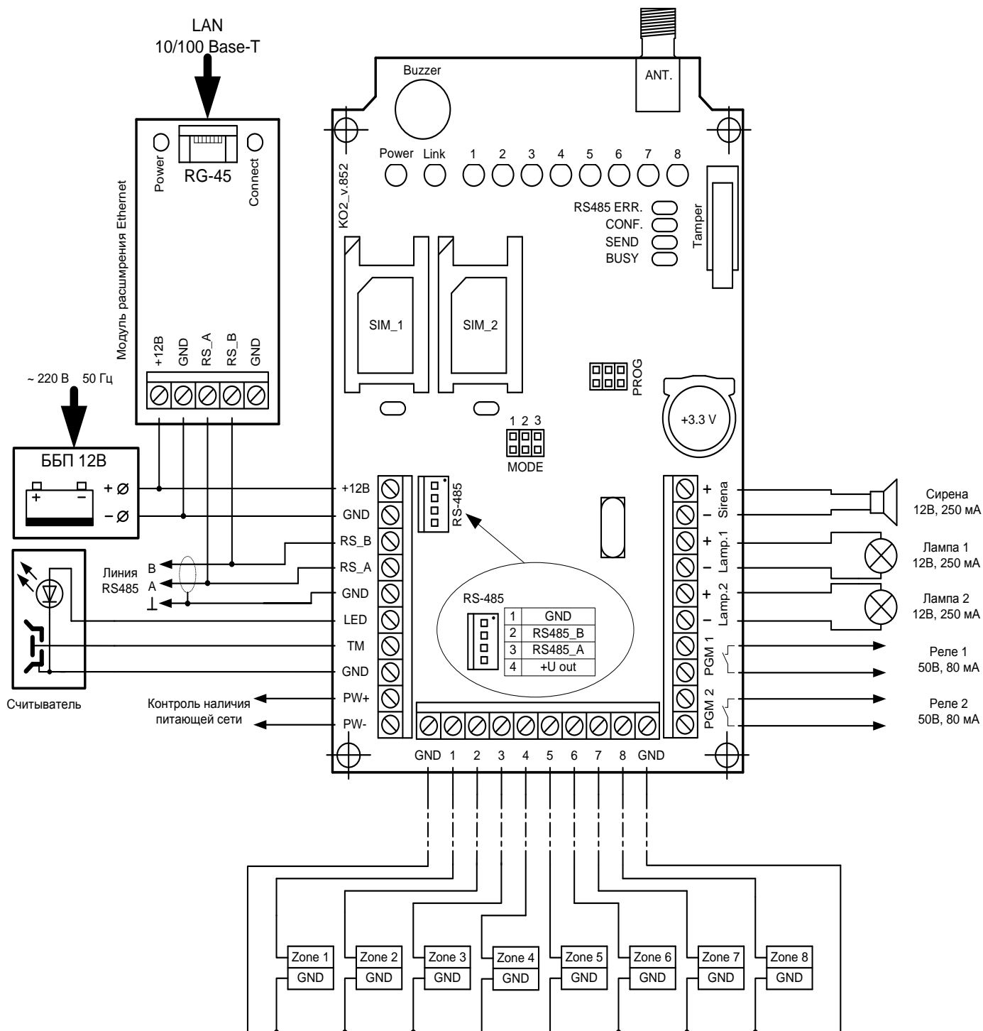
Рисунок 3. Схема подключения прибора.
