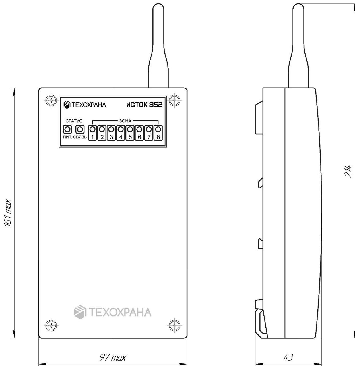
Рисунок 1. Габаритные размеры УОО «ИСТОК 852»
