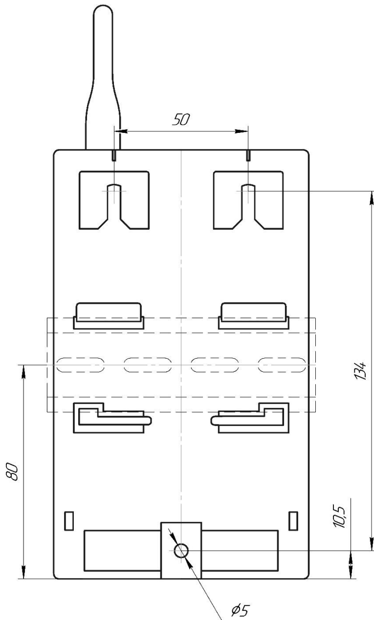
Рисунок 2. Установочные размеры УОО «ИСТОК 852».
