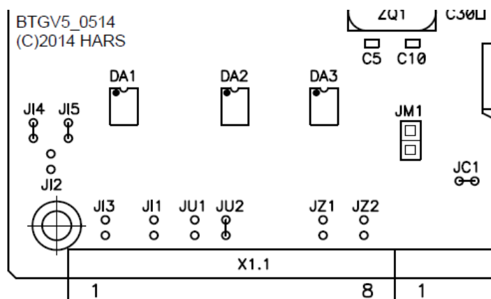
Рис.3. Контроллер BTGV5_0514. Расположение переключателей для универсального варианта.
