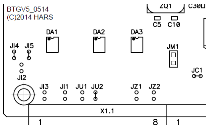
Рис.3. Контроллер BTGV5_0514. Расположение перемычек для универсального варианта.
